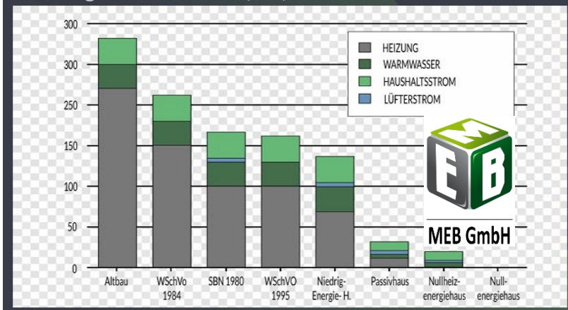
Endenergiekennwert kWh/(m²a)
